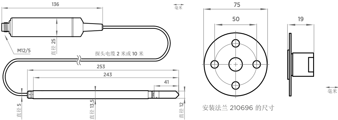
HMP5 探头尺寸
