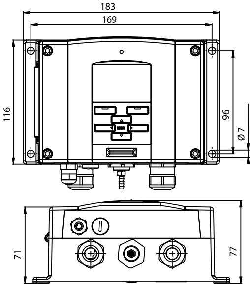
尺寸 (mm)
